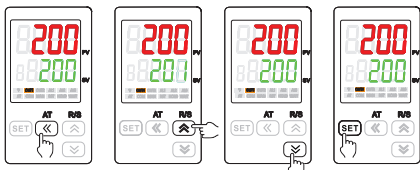
短按“SET”键SV值闪烁 短按“R/S”键增加SV值 短按“S”键减少SV值 短按“SET”键保存SV值
