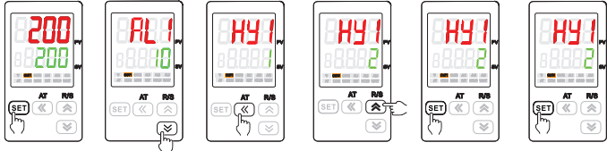
长按“SET”键3秒进入常用菜单 短按“R/S”或“S”键切换菜单 短按“S”键参数闪烁 短按“R/S”或“S”键修改参数 短按“SET”键保存参数 长按“SET”键3秒退出菜单
